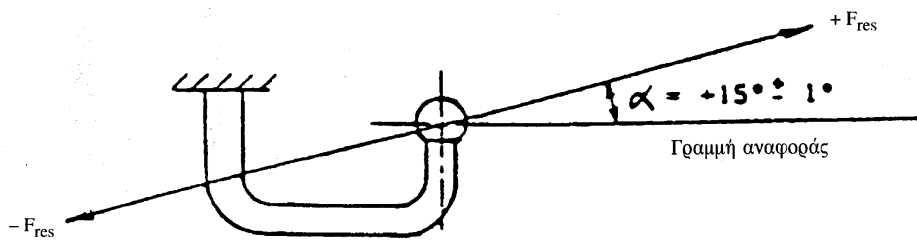
Σχήμα 18 Διάταξη δοκιμής II
